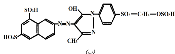
شکل ۸ - رنگ‌های راکتیو مناسب استتار برای الیاف ویسکوز ریون رنگری جرمی شده با CB [۵۱].
