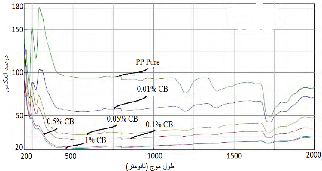
شکل ۱۷- طیف‌های انعکاسی نخ فیلامنتی خالص و اصلاح شده پلی پروپیلین با استفاده از کربن سیاه با ابعاد ذره نانو با مقادیر متفاوت [۳۹].
